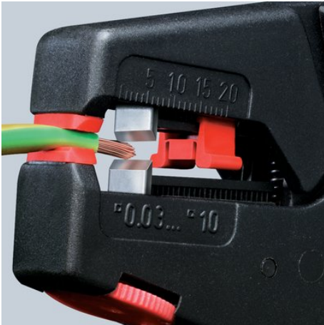
12 40 200: dezizolare de precizie, fără deteriorarea conductorului
